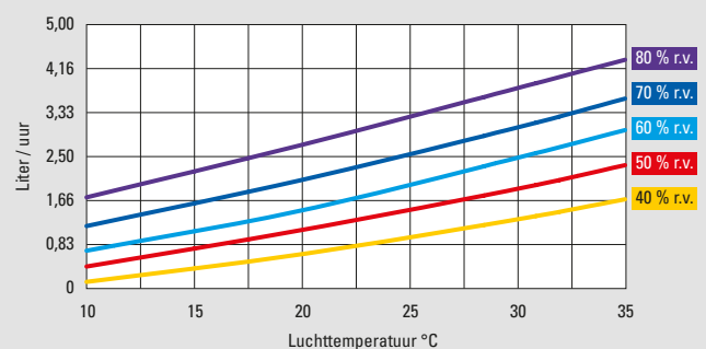
Ontvochtigingscapaciteit DS 60
