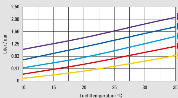
Ontvochtigingscapaciteit DS 30
